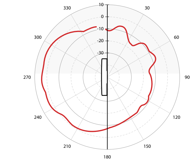
BLE Vertical
