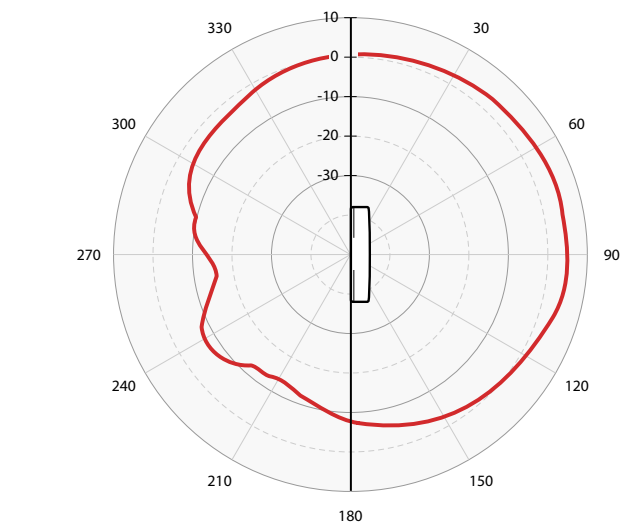
BLE Horizontal
